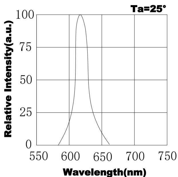
相对发光强度与波长 (Ta=25℃)
