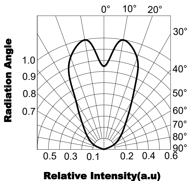
角度与相对发光强度 (Ta=25℃)
