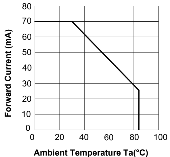
最大正向电流与环境温度
