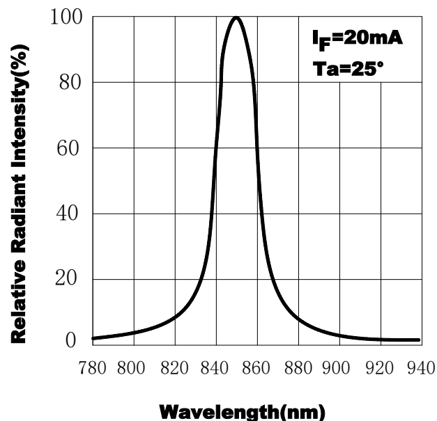
图.2 频谱分布
