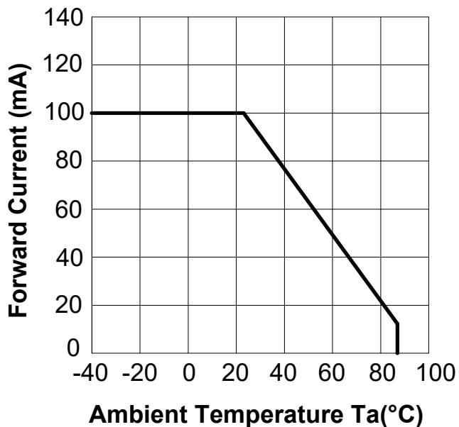
图.1 正向电流与环境温度
