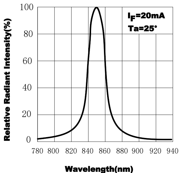
图.2 频谱分布
