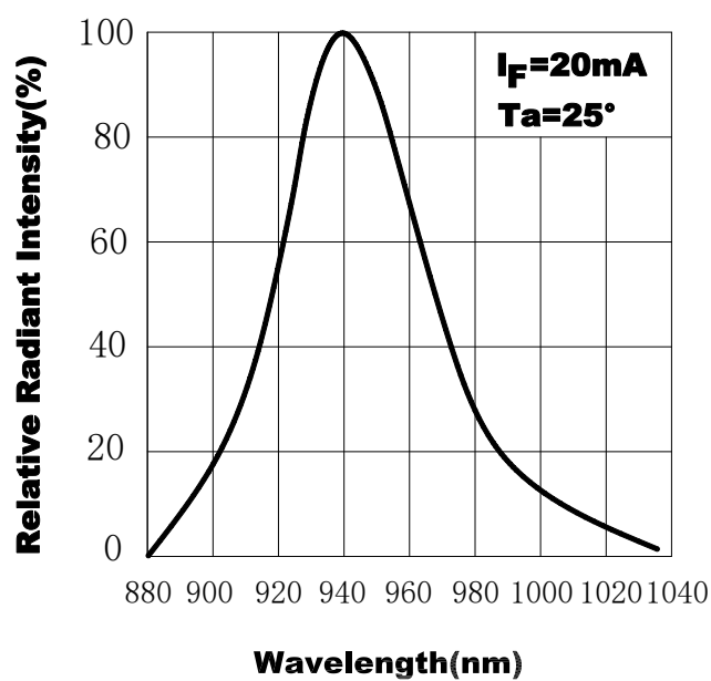
图.2 频谱分布
