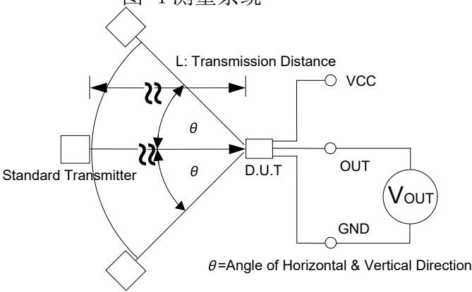
图-4 测量系统
