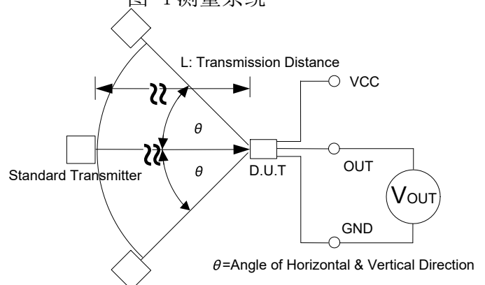
图-4 测量系统
